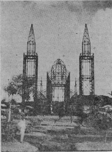
Armazón de acero de la Iglesia de San Ramón cuyos trabajos dirige el Ingeniero don Hernán Gutiérrez
